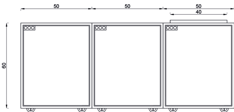
ÖN GÖRÜNÜŞ-1
